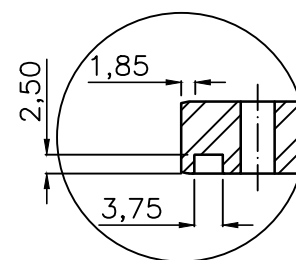
DETALHE R ESCALA 1:1
